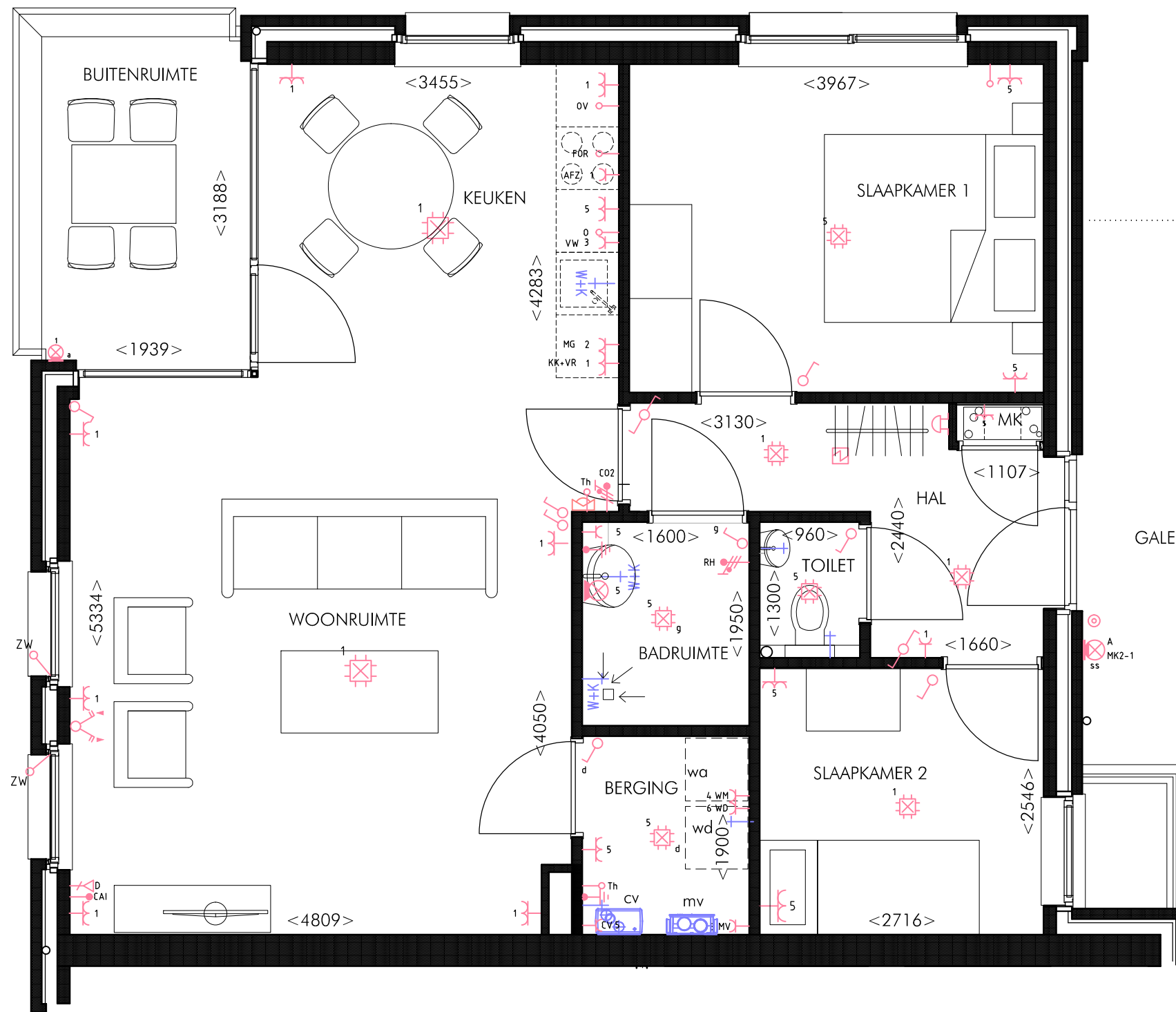
1E VERDIEPING TYPE A1
