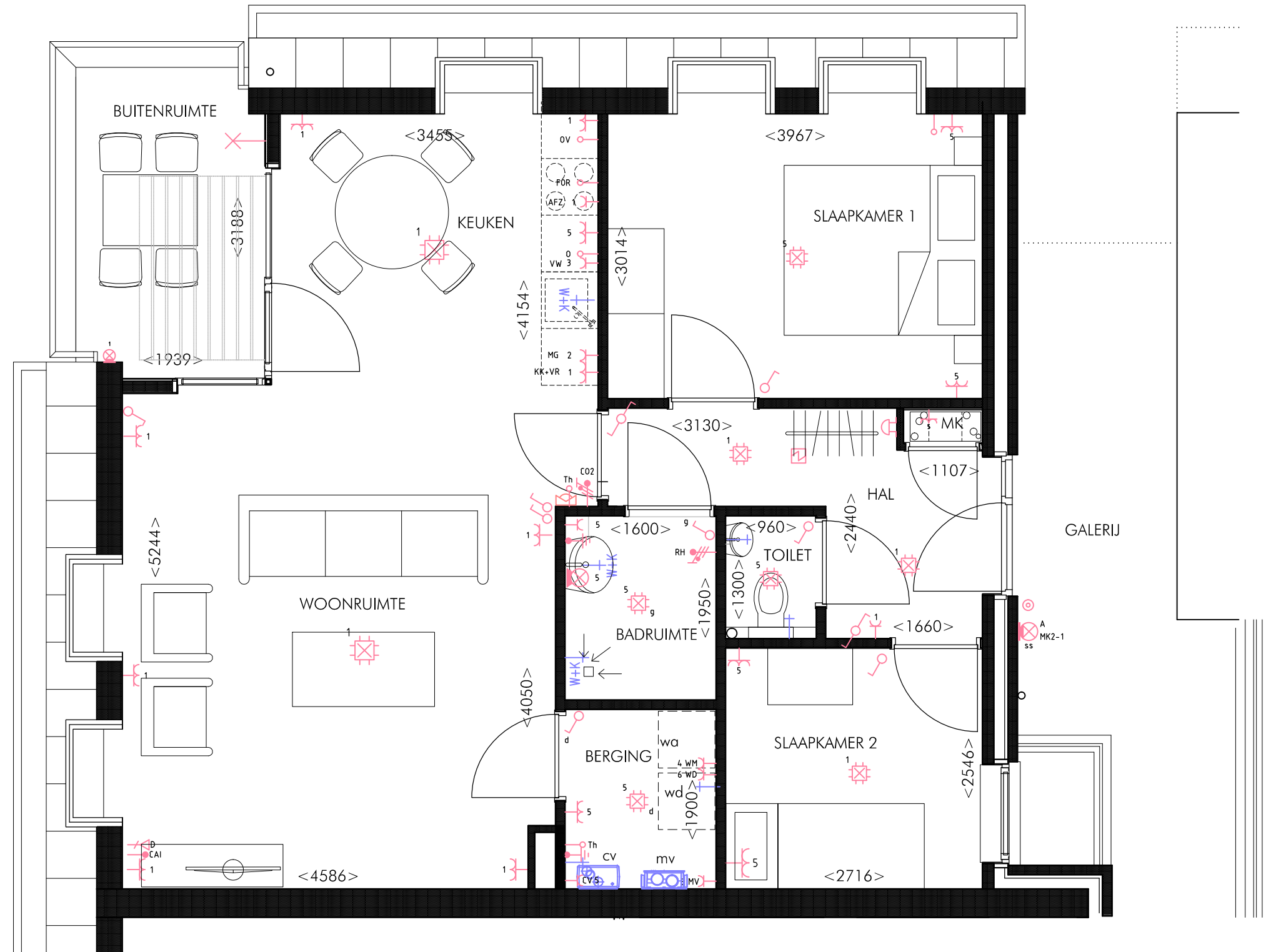
2E VERDIEPING TYPE A1
